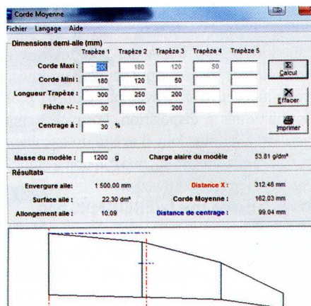
«Corde Moyenne» est l'utilitaire à installer sur son PC! Il facilite les calculs de centrage des ailes complexes.
